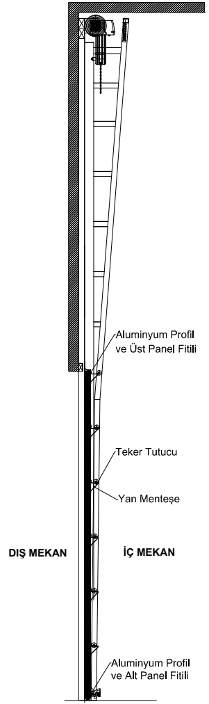
B - B KESİTİ
